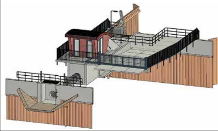
3D-ontwerp van het nieuwe vijzelgemaal dat nu aan de oostkant van de Trekvaart wordt gemaakt.
